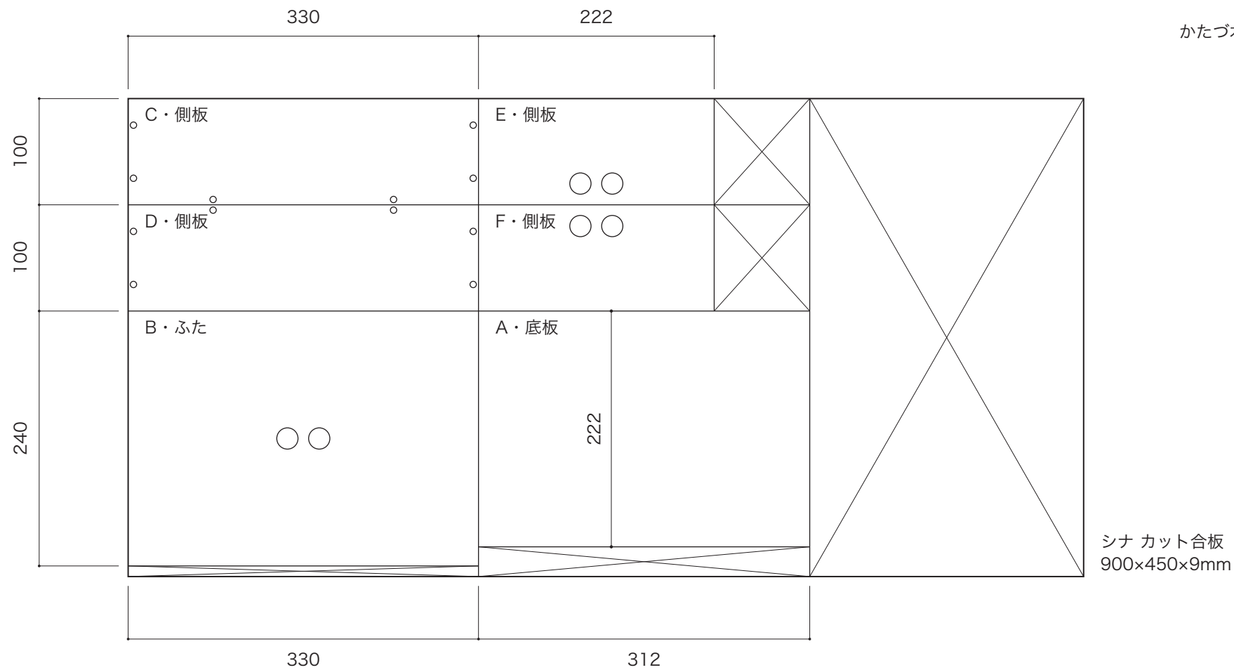
ねじをうつ位置
