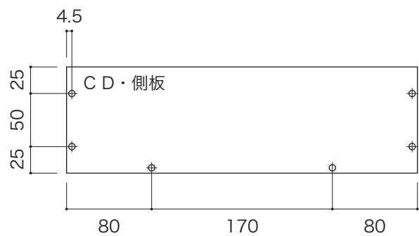
ねじをうつ位置
