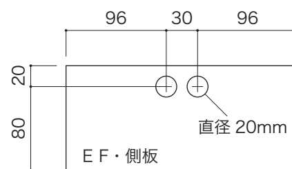
もち手となる穴をあける位置
